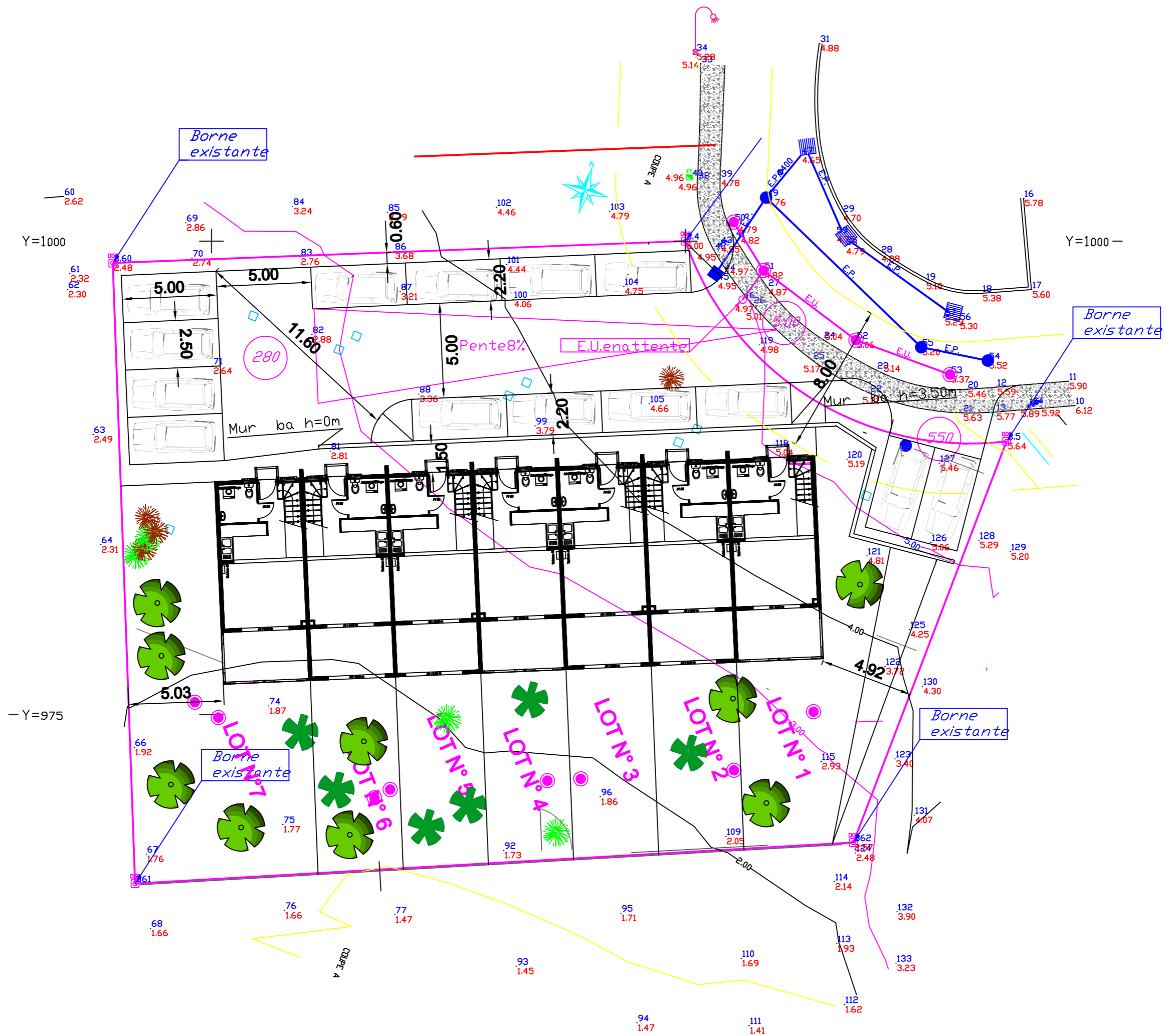
LES CLOS DE BETANIA Plan Masse du 13 Janvier 2017
